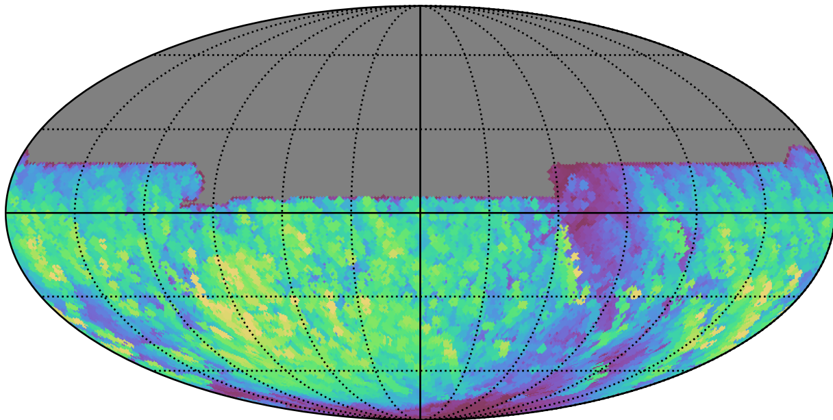
weather_cloudso18v3.4_10yrs All sky y band: Max normairmass
