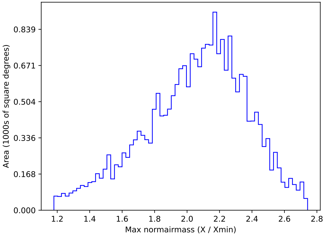
weather_cloudso18v3.4_10yrs All sky y band: Max normairmass
