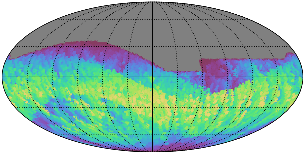
weather_cloudso18v3.4_10yrs All sky i band: Max normairmass
