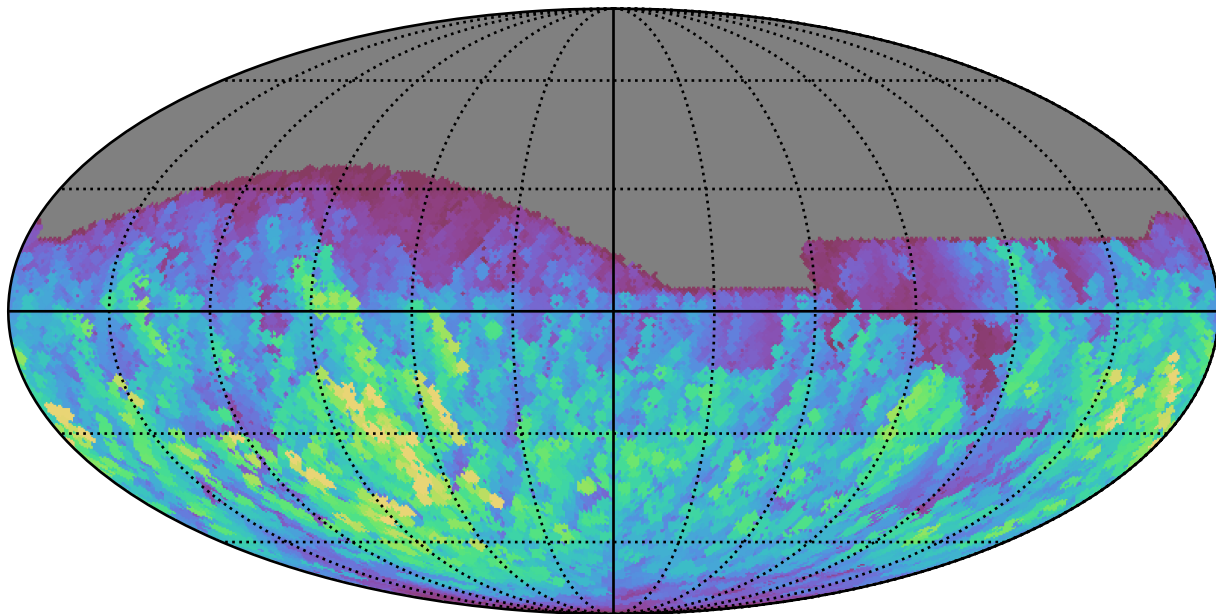
weather_cloudso18v3.4_10yrs All sky g band: Max normairmass
