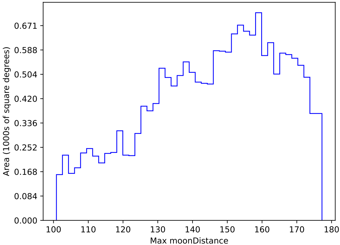
weather_cloudso18v3.4_10yrs WFD y band: Max moonDistance
