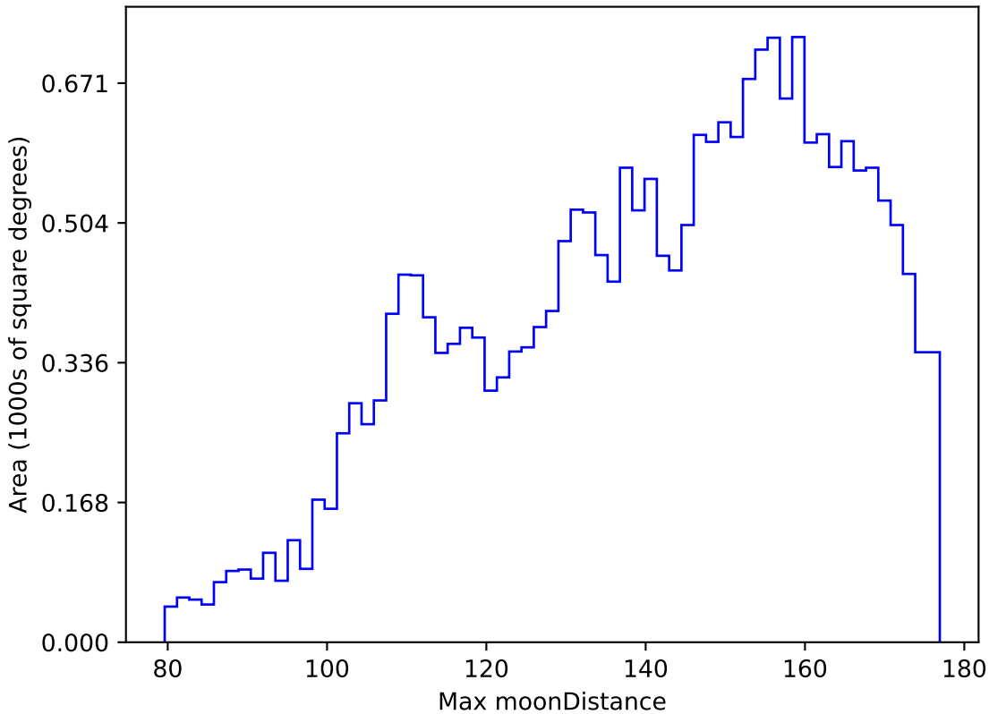
weather_cloudso18v3.4_10yrs All sky y band: Max moonDistance
