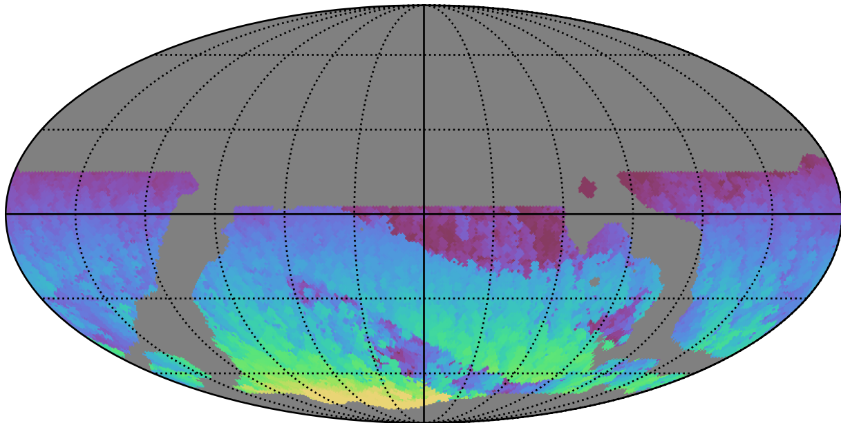
weather_cloudso18v3.4_10yrs WFD z band: Max HA
