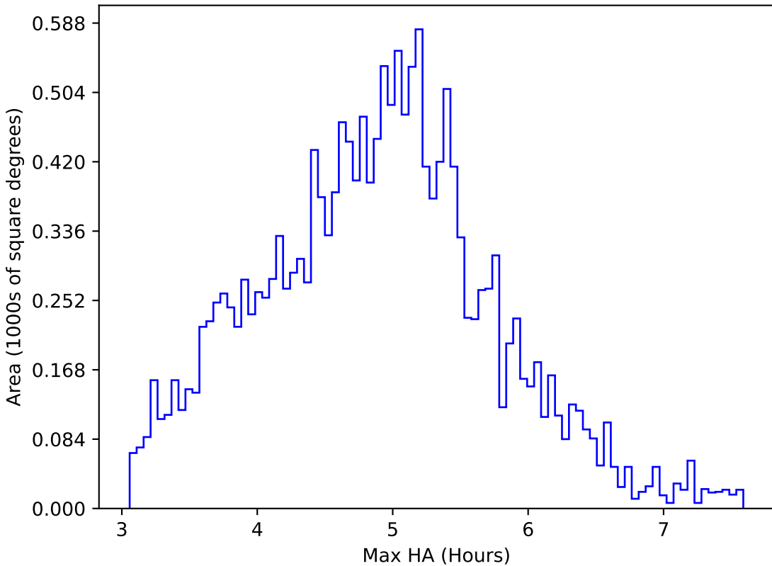
weather_cloudso18v3.4_10yrs WFD z band: Max HA
