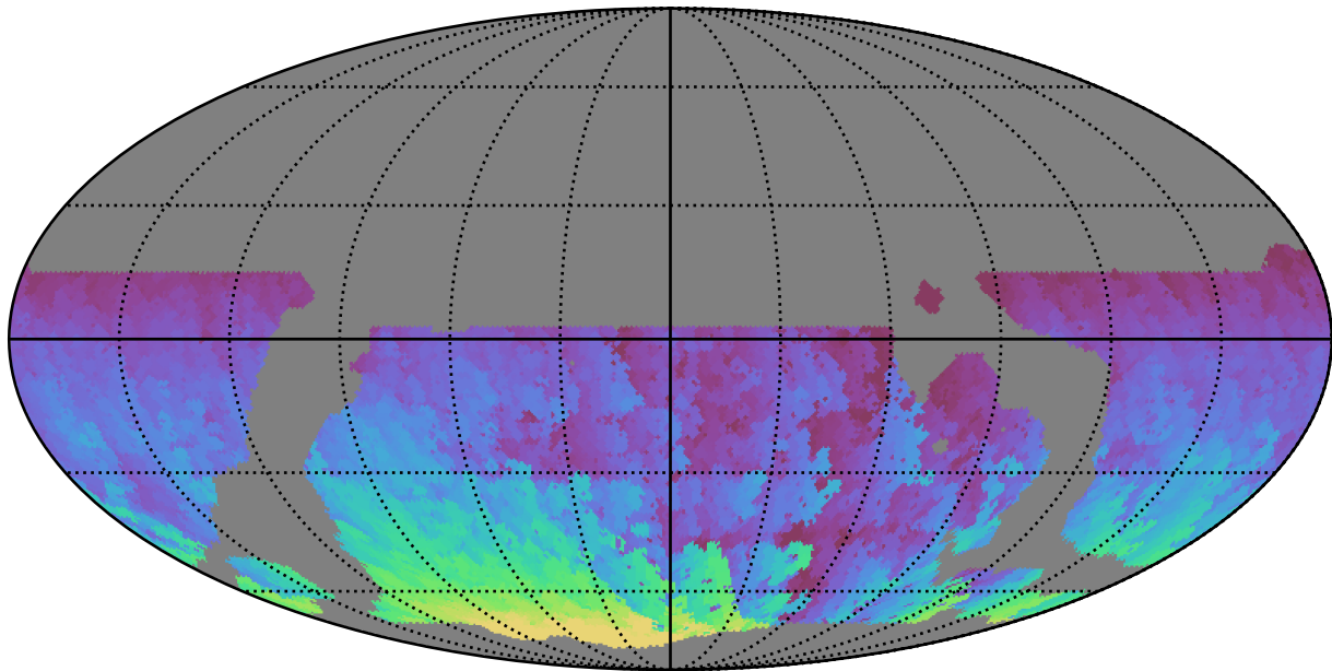
weather_cloudso18v3.4_10yrs WFD y band: Max HA
