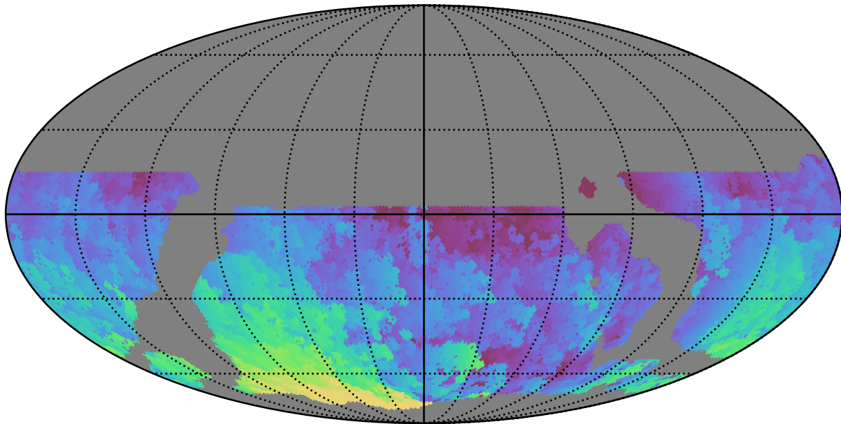
weather_cloudso18v3.4_10yrs WFD u band: Max HA
