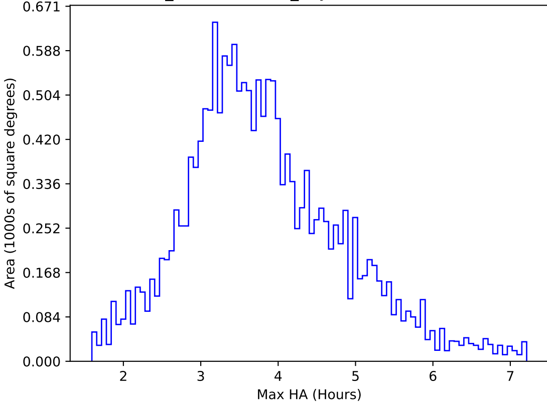
weather_cloudso18v3.4_10yrs WFD u band: Max HA
