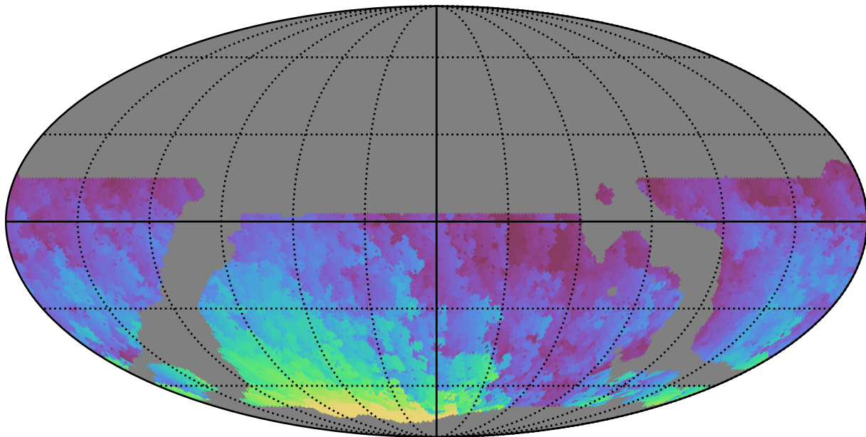
weather_cloudso18v3.4_10yrs WFD r band: Max HA
