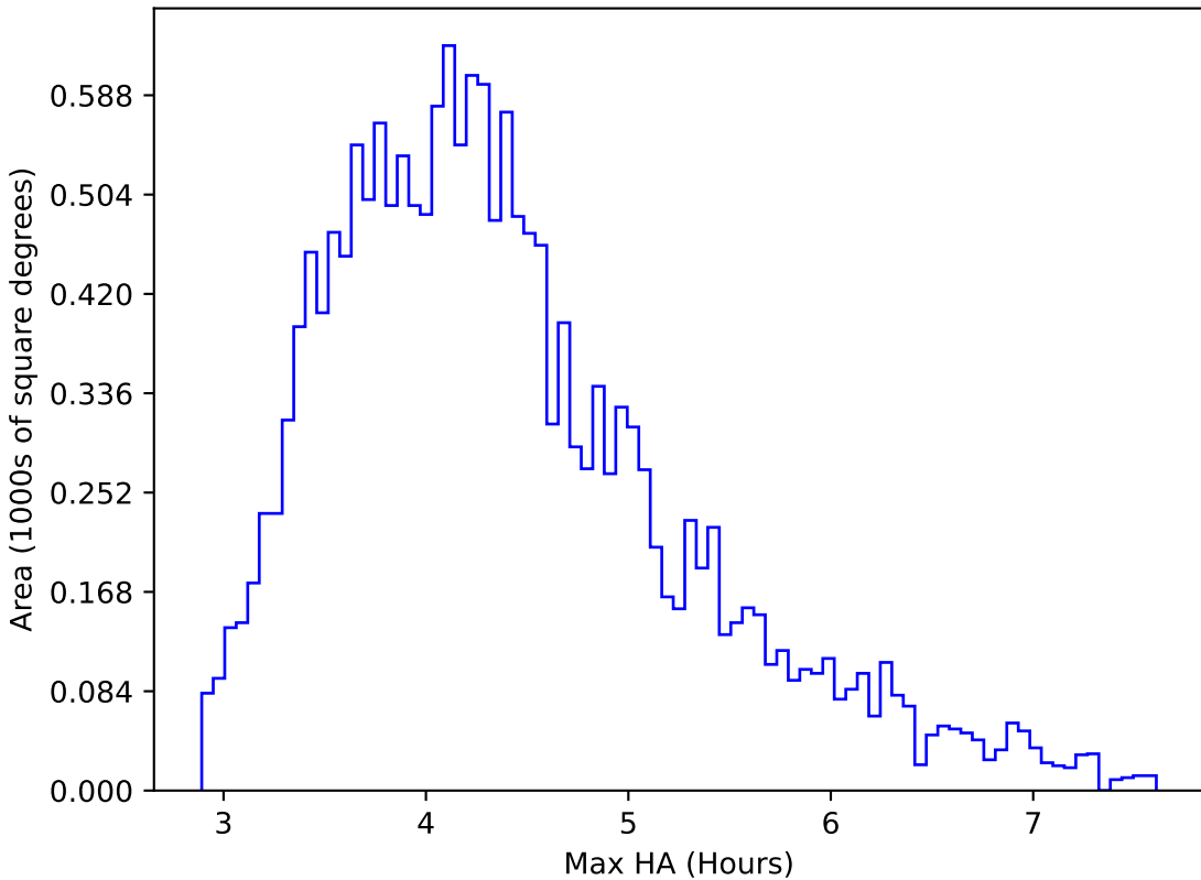
weather_cloudso18v3.4_10yrs WFD r band: Max HA
