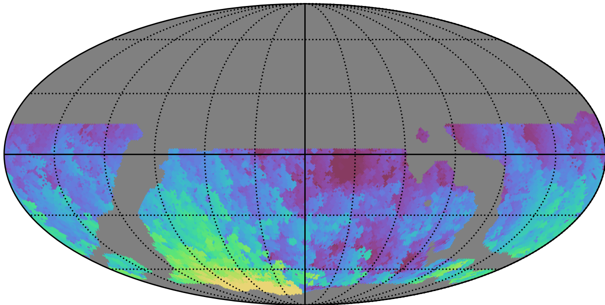
weather_cloudso18v3.4_10yrs WFD g band: Max HA
