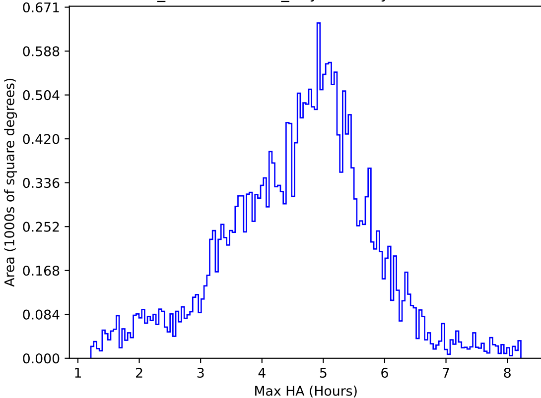
weather_cloudso18v3.4_10yrs All sky z band: Max HA
