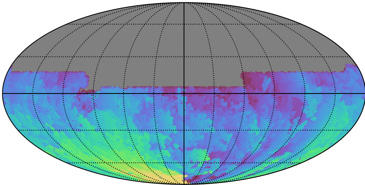
weather_cloudso18v3.4_10yrs All sky u band: Max HA
