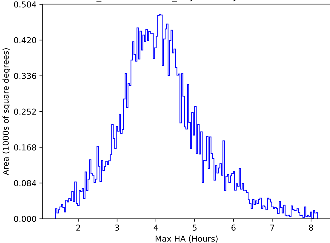
weather_cloudso18v3.4_10yrs All sky r band: Max HA
