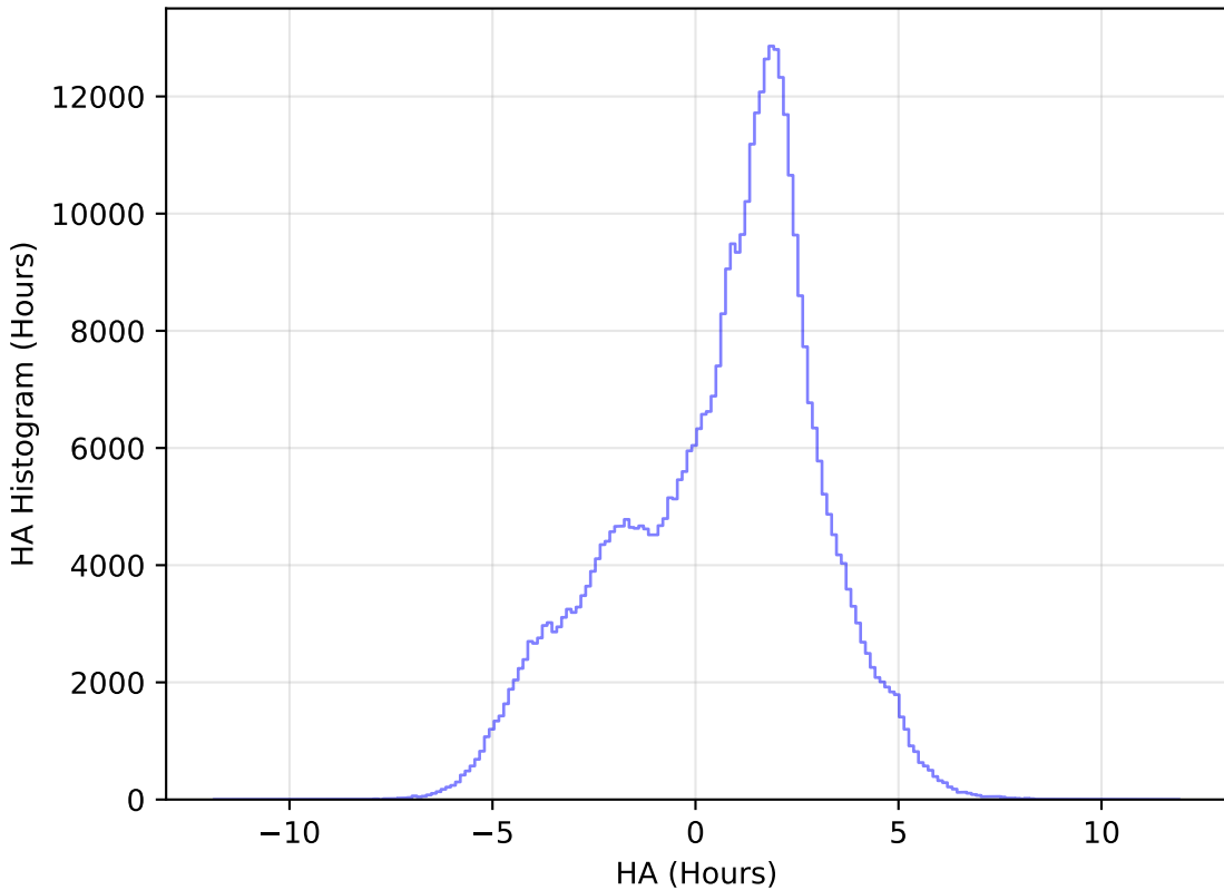
weather_cloudso18v3.4_10yrs WFD z band: HA Histogram
