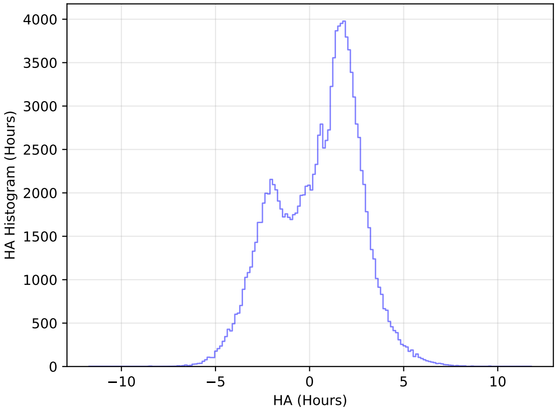
weather_cloudso18v3.4_10yrs WFD u band: HA Histogram
