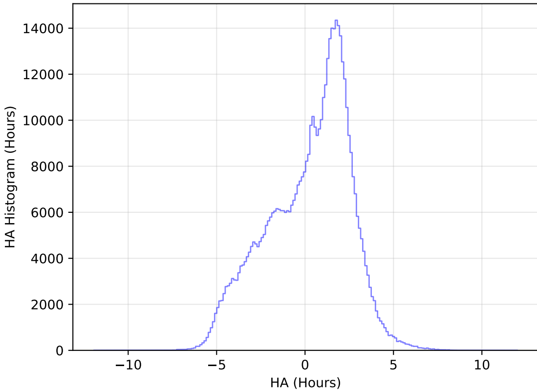
weather_cloudso18v3.4_10yrs WFD r band: HA Histogram
