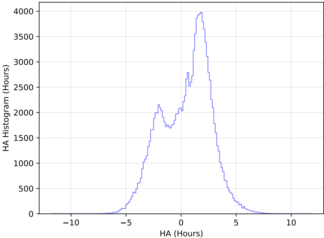
weather_cloudso18v3.4_10yrs All sky u band: HA Histogram
