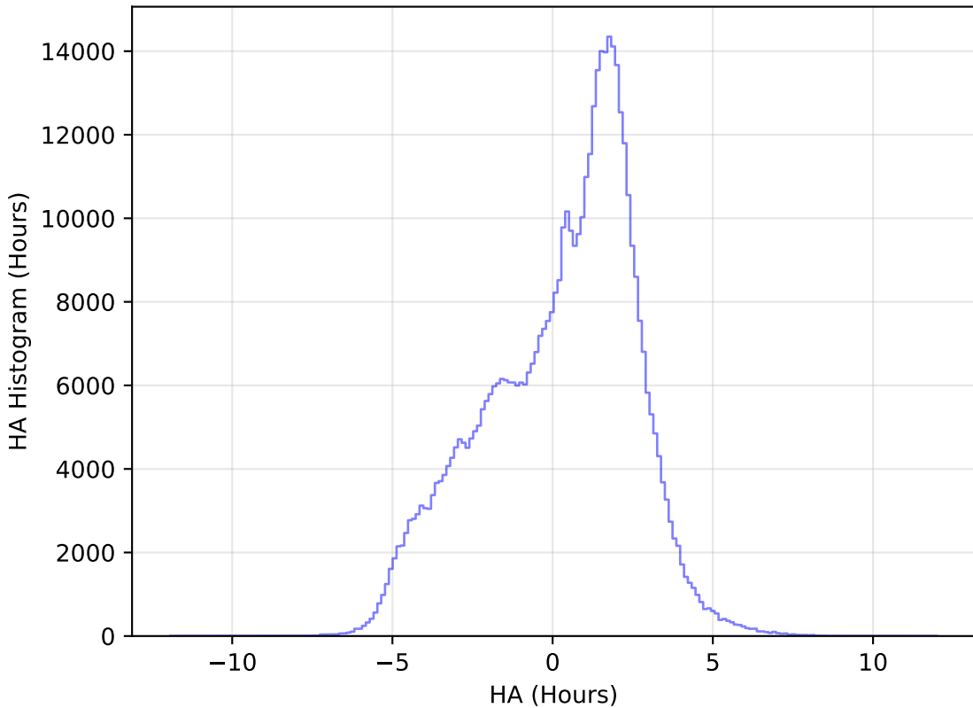
weather_cloudso18v3.4_10yrs All sky r band: HA Histogram
