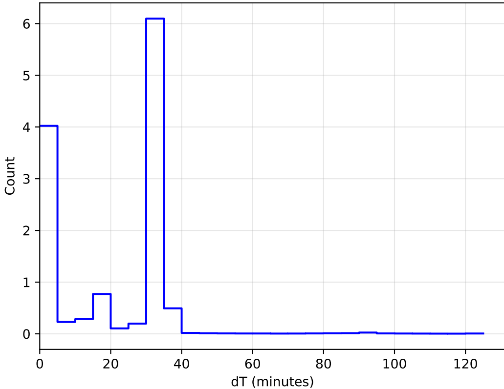
weather_cloudso18v3.4_10yrs WFD: DeltaT Histogram
