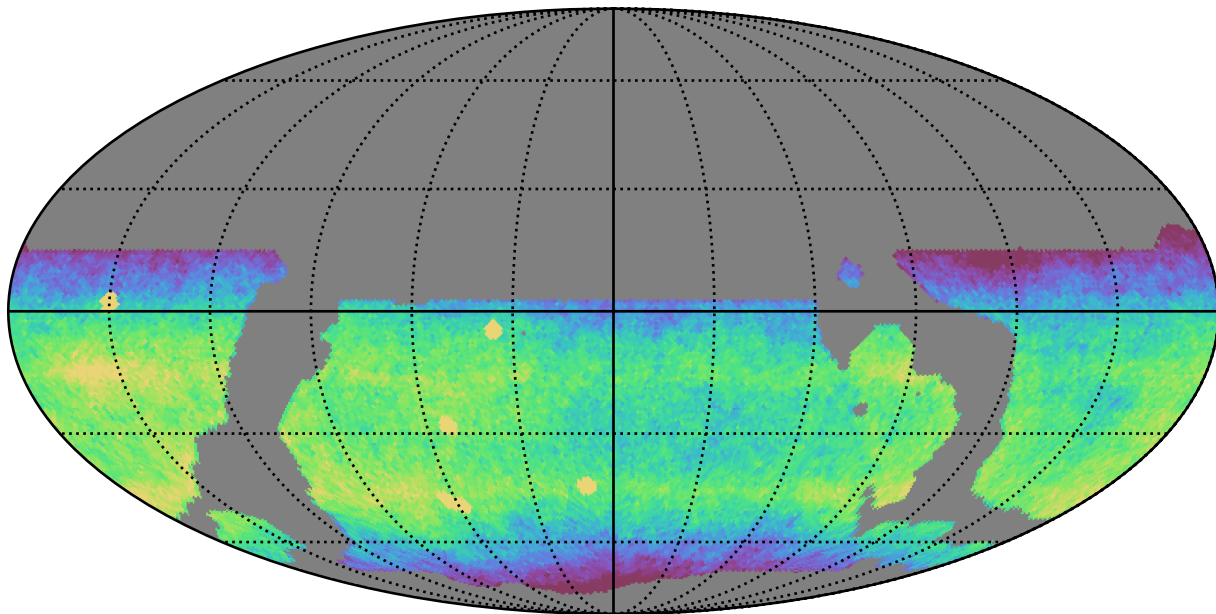
weather_cloudso18v3.4_10yrs WFD i band: CoaddM5
