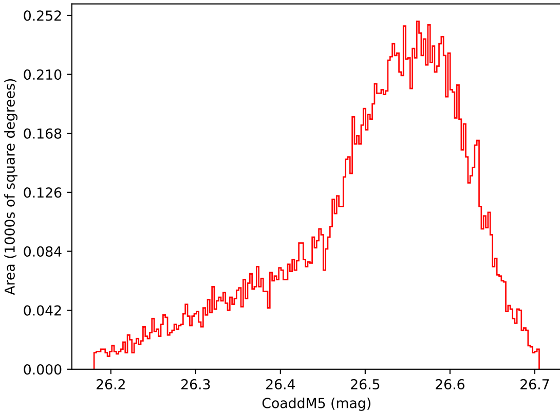
weather_cloudso18v3.4_10yrs WFD i band: CoaddM5
