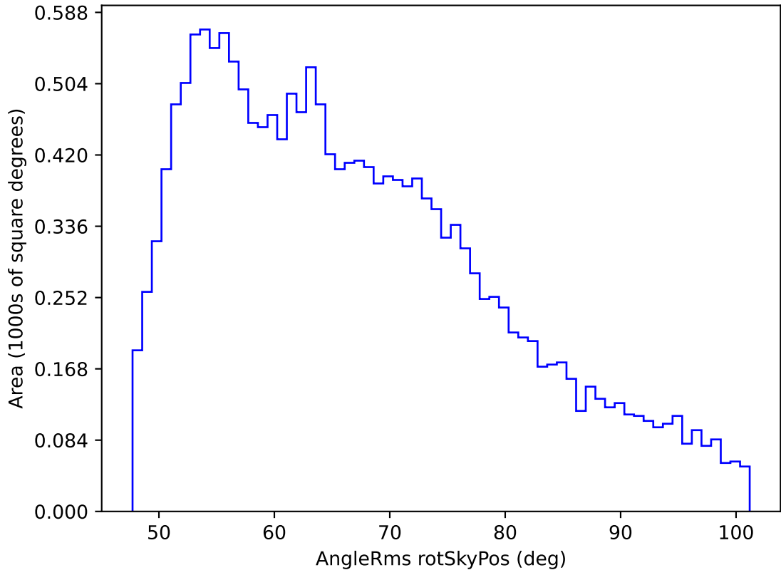
weather_cloudso18v3.4_10yrs WFD z band: AngleRms rotSkyPos
