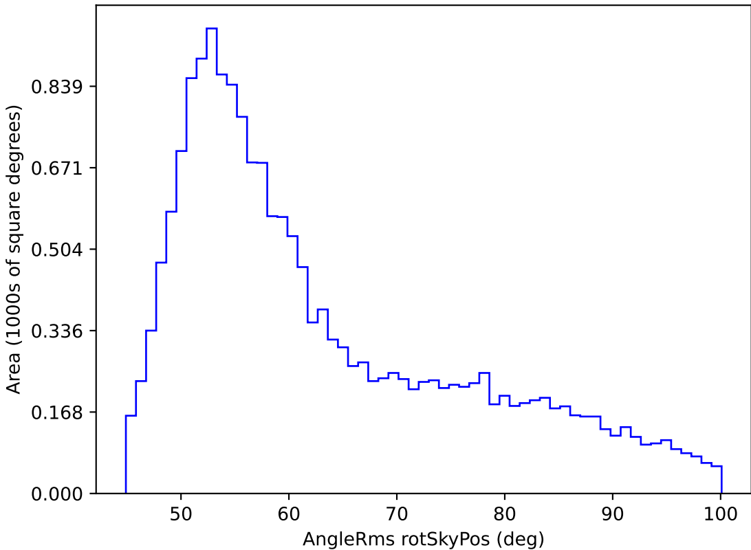
weather_cloudso18v3.4_10yrs WFD u band: AngleRms rotSkyPos
