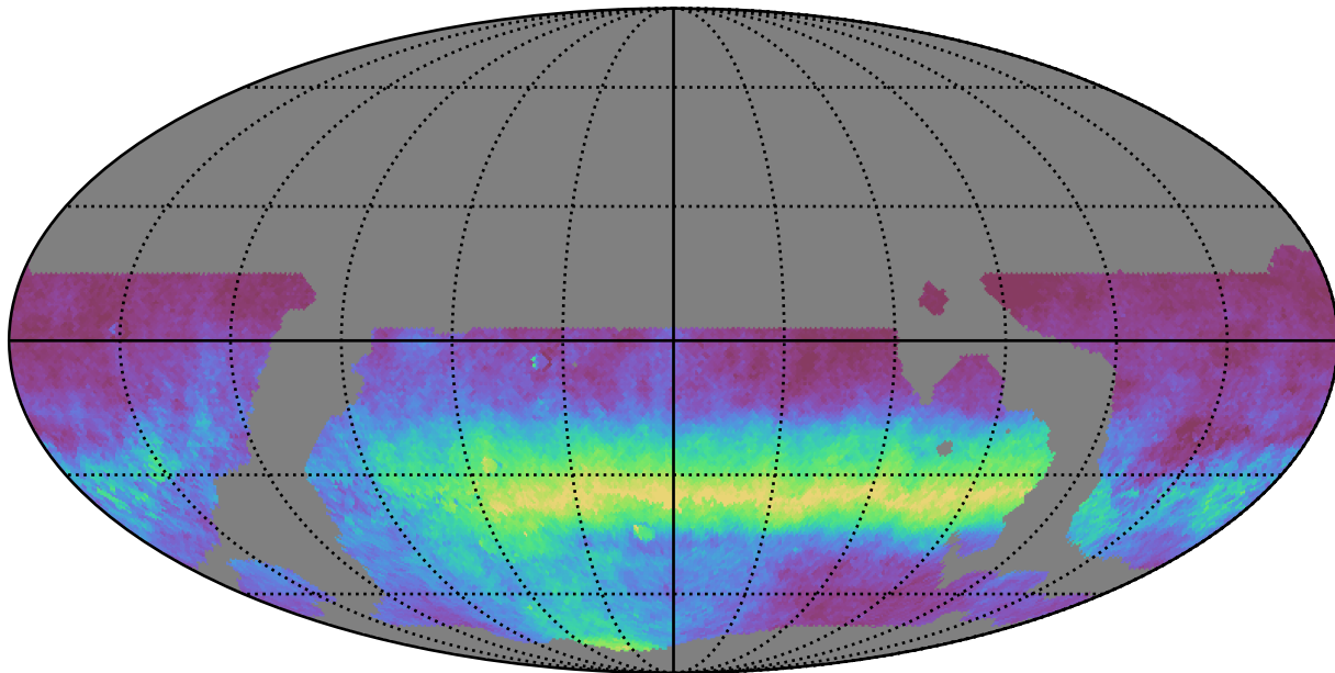
weather_cloudso18v3.4_10yrs WFD r band: AngleRms rotSkyPos
