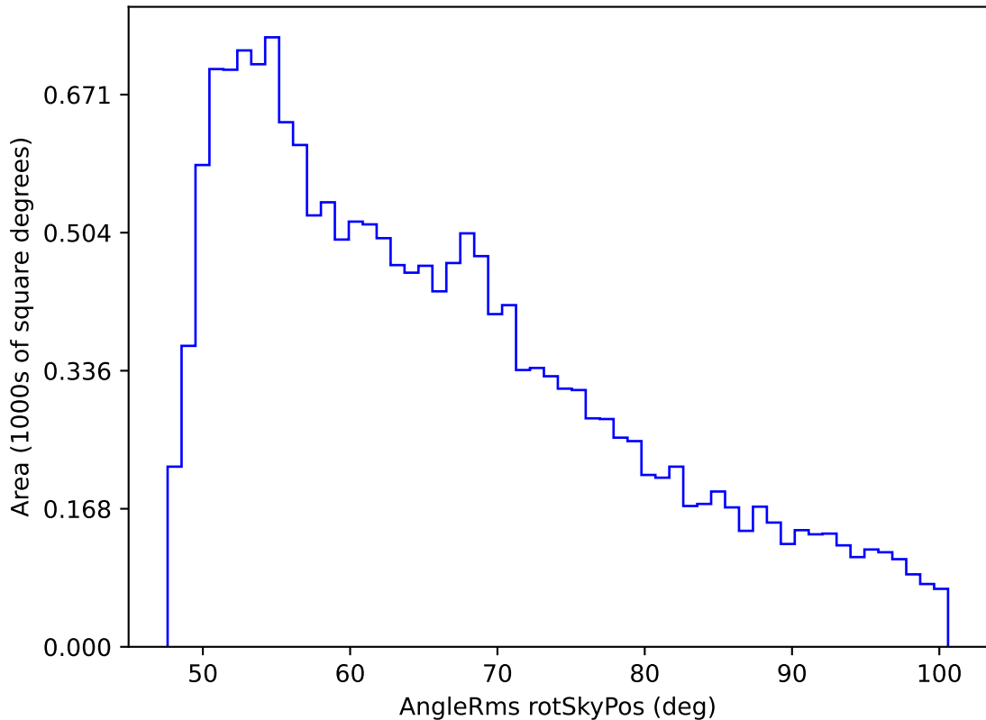
weather_cloudso18v3.4_10yrs WFD r band: AngleRms rotSkyPos
