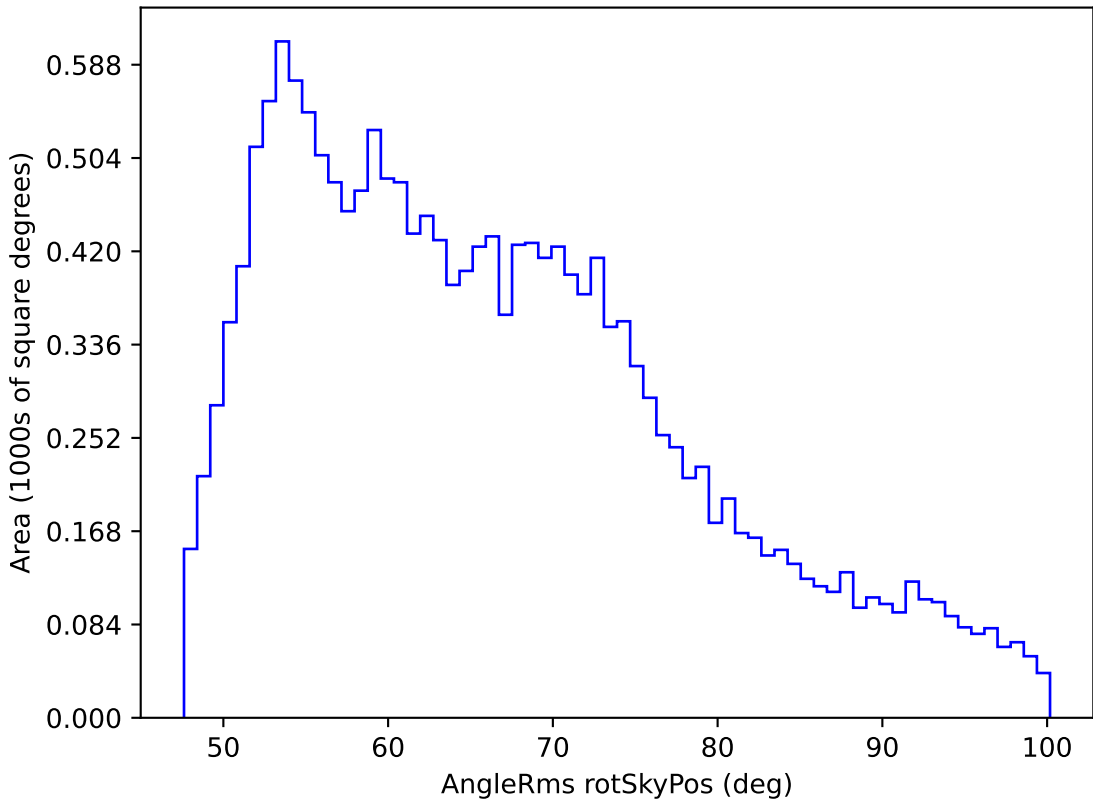
weather_cloudso18v3.4_10yrs WFD i band: AngleRms rotSkyPos
