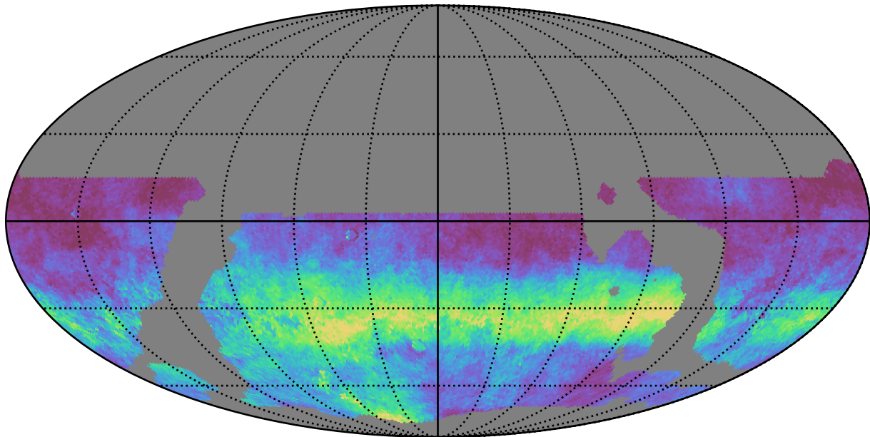
weather_cloudso18v3.4_10yrs WFD g band: AngleRms rotSkyPos
