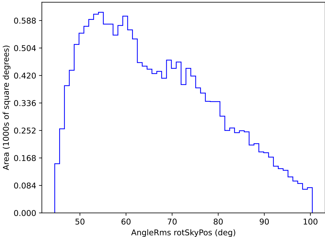
weather_cloudso18v3.4_10yrs WFD g band: AngleRms rotSkyPos
