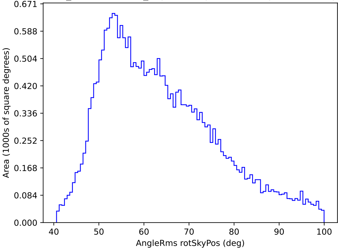
weather_cloudso18v3.4_10yrs All sky z band: AngleRms rotSkyPos
