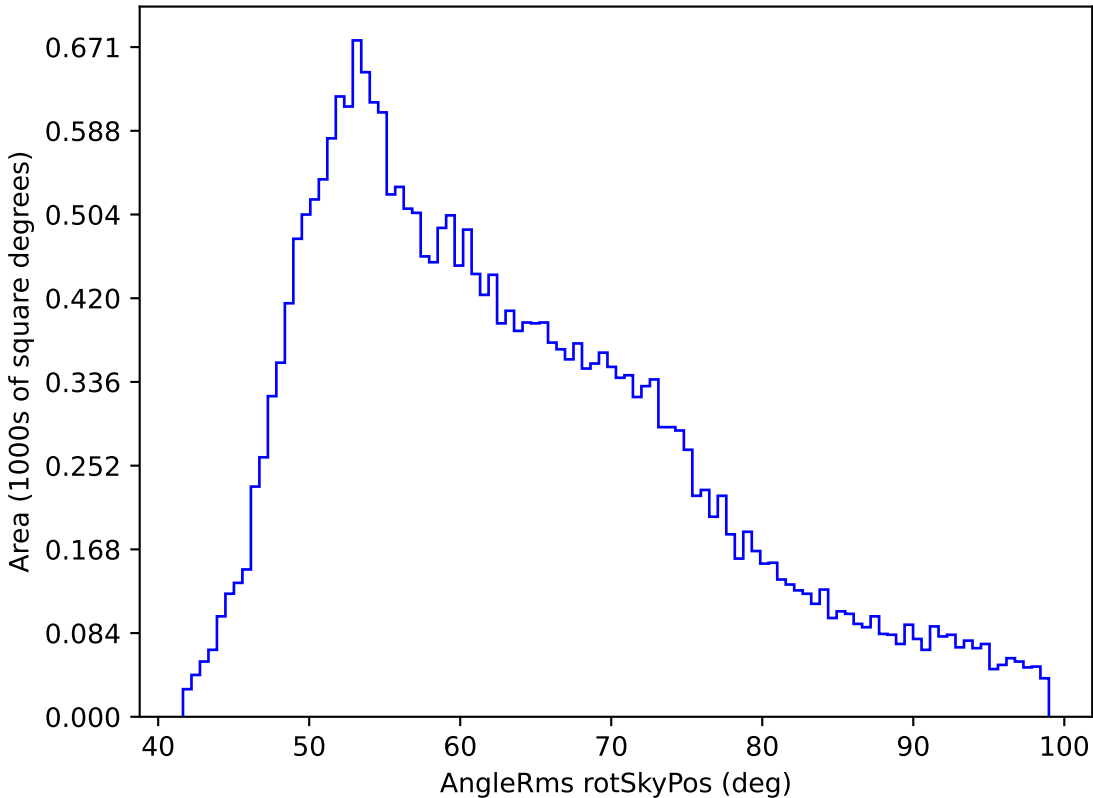
weather_cloudso18v3.4_10yrs All sky i band: AngleRms rotSkyPos
