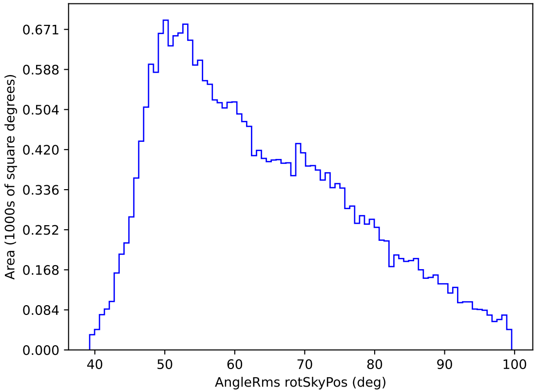
weather_cloudso18v3.4_10yrs All sky g band: AngleRms rotSkyPos
