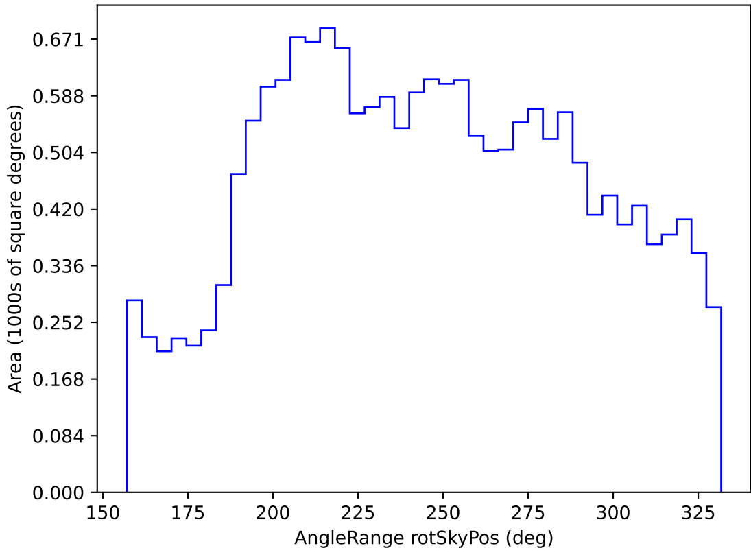
weather_cloudso18v3.4_10yrs WFD u band: AngleRange rotSkyPos
