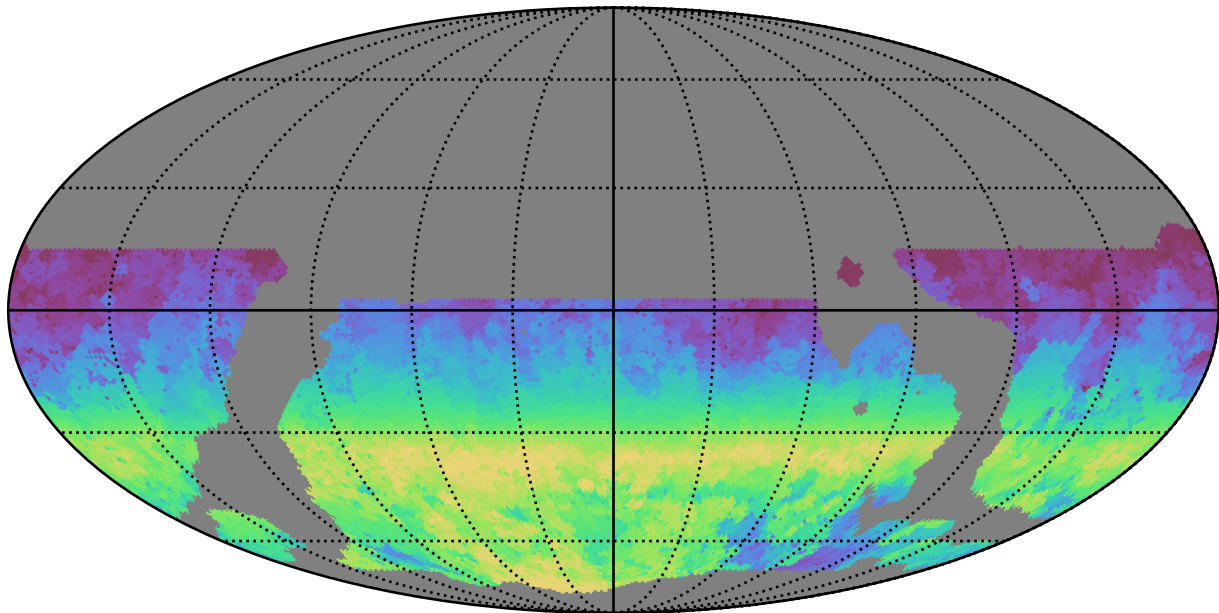
weather_cloudso18v3.4_10yrs WFD r band: AngleRange rotSkyPos
