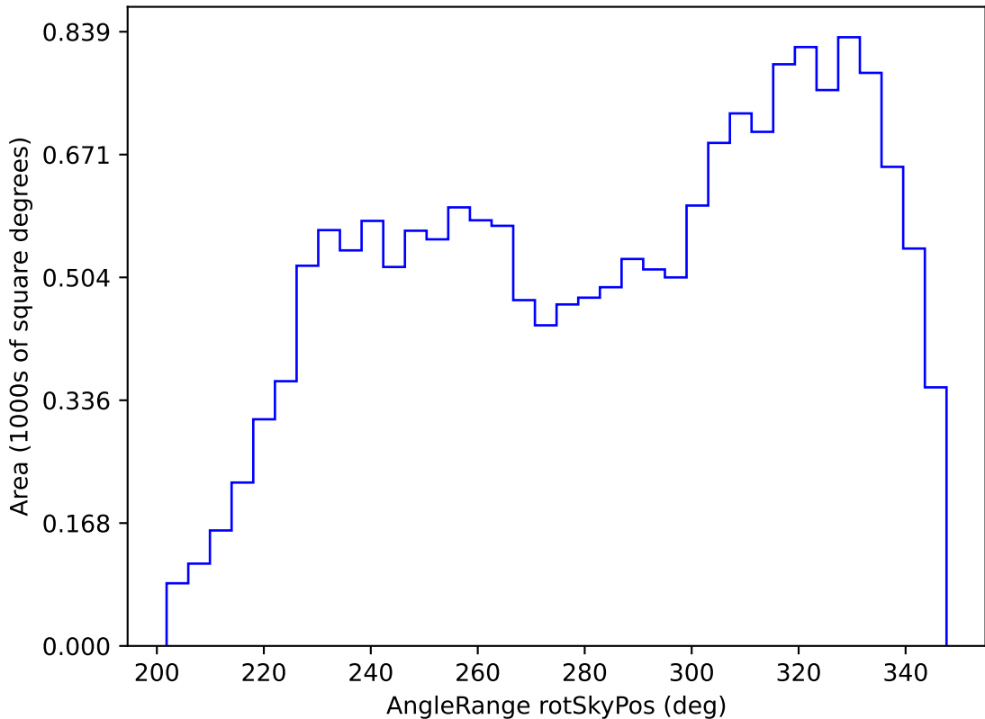
weather_cloudso18v3.4_10yrs WFD i band: AngleRange rotSkyPos
