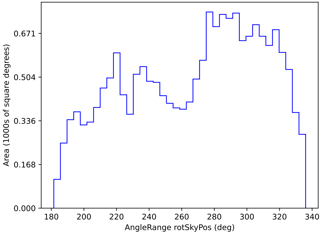
weather_cloudso18v3.4_10yrs WFD g band: AngleRange rotSkyPos
