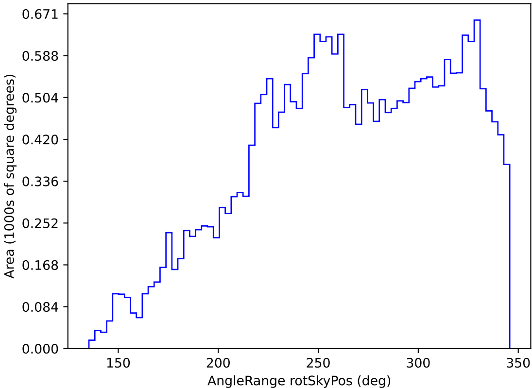
weather_cloudso18v3.4_10yrs All sky z band: AngleRange rotSkyPos
