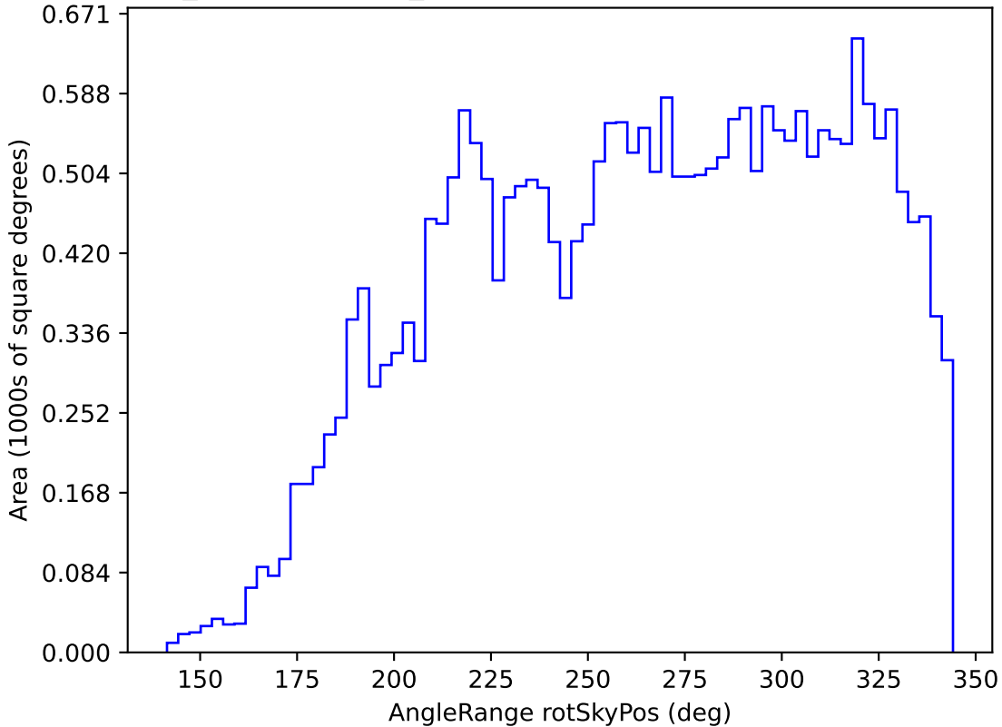
weather_cloudso18v3.4_10yrs All sky r band: AngleRange rotSkyPos
