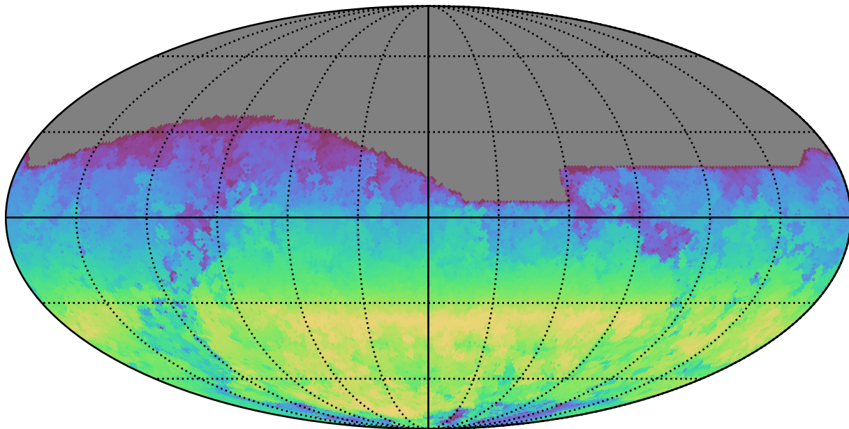
weather_cloudso18v3.4_10yrs All sky i band: AngleRange rotSkyPos
