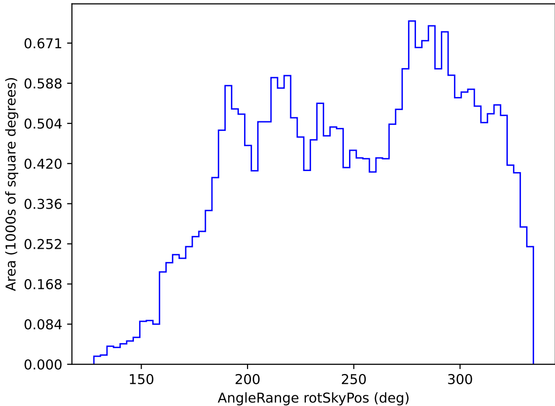
weather_cloudso18v3.4_10yrs All sky g band: AngleRange rotSkyPos
