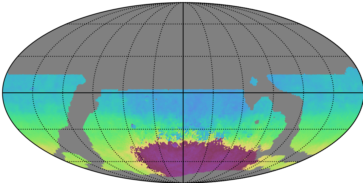
weather_cloudso18v3.4_10yrs WFD y band: AngleMean rotSkyPos
