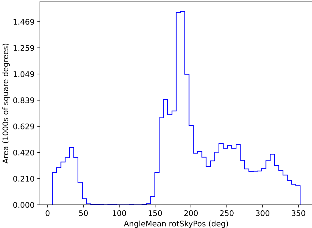
weather_cloudso18v3.4_10yrs WFD y band: AngleMean rotSkyPos
