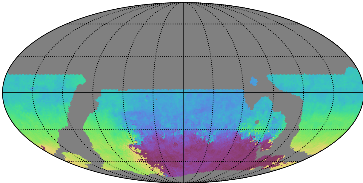
weather_cloudso18v3.4_10yrs WFD u band: AngleMean rotSkyPos
