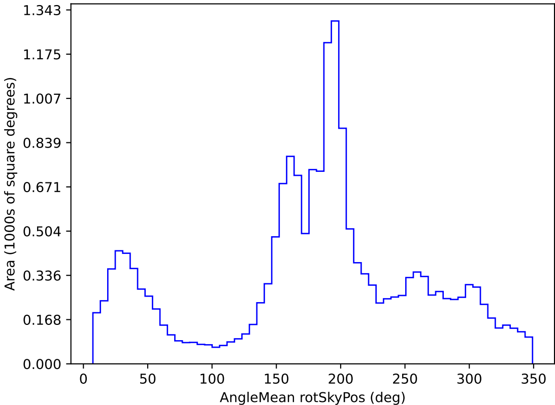
weather_cloudso18v3.4_10yrs WFD u band: AngleMean rotSkyPos
