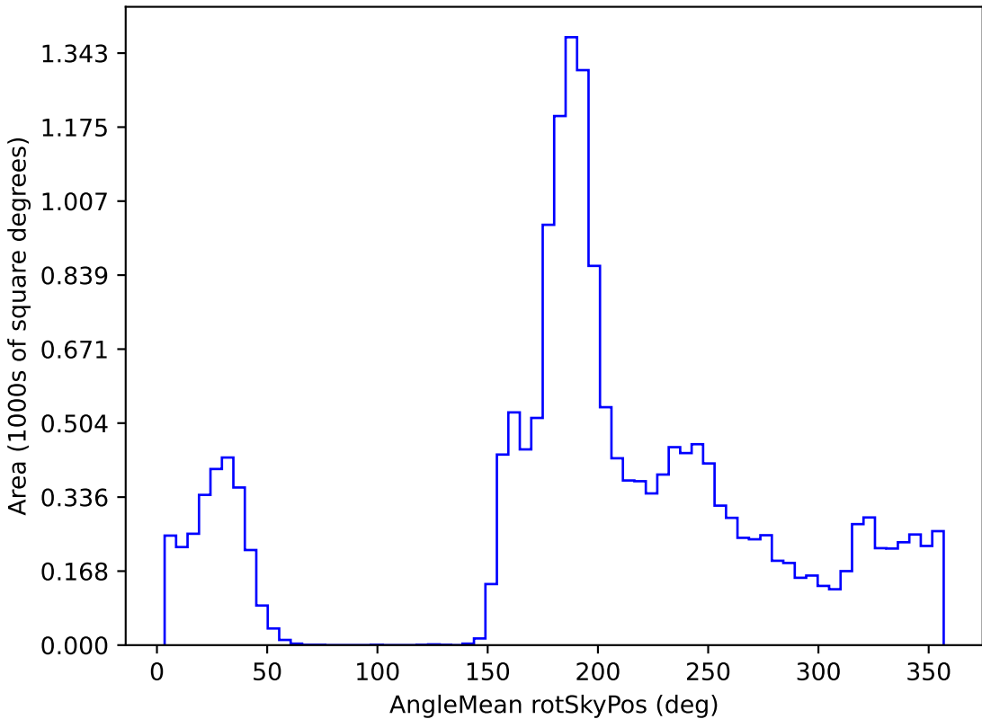
weather_cloudso18v3.4_10yrs WFD i band: AngleMean rotSkyPos
