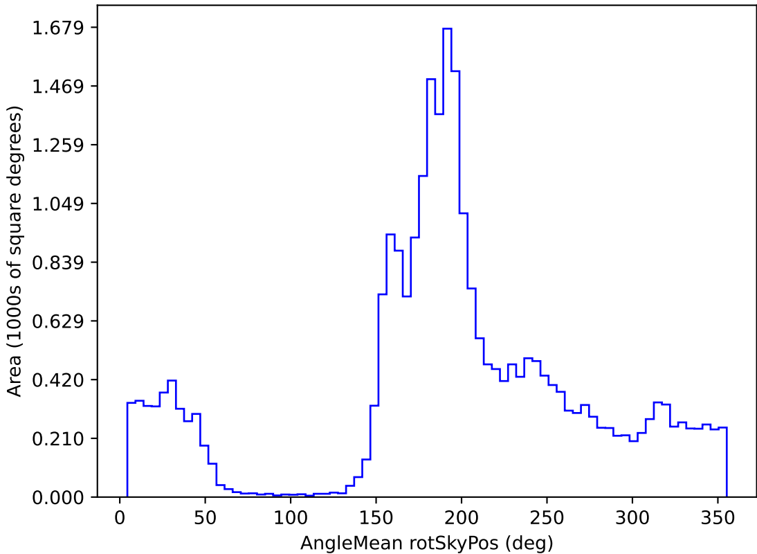
weather_cloudso18v3.4_10yrs All sky z band: AngleMean rotSkyPos
