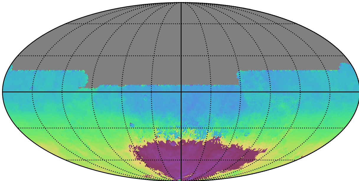
weather_cloudso18v3.4_10yrs All sky y band: AngleMean rotSkyPos
